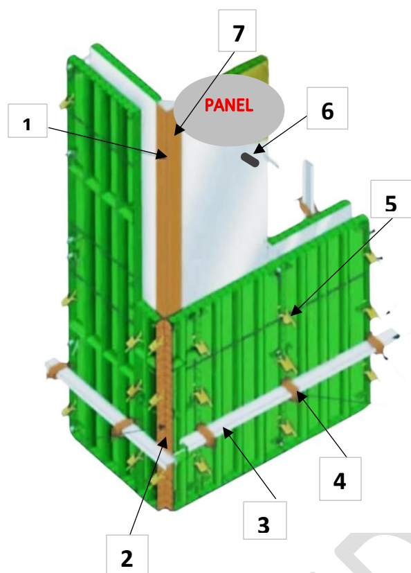
FORMALETA COLUMNA COMPLETA DIVIDIDA EN 2 PARTES
